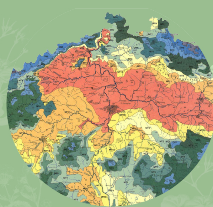
Mapa klimatických oblastí
